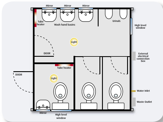
2 Plus 1 Toilet block layout
